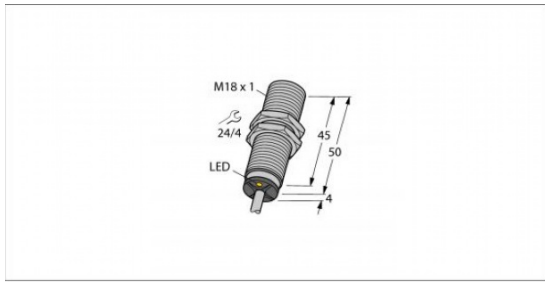
BI5-M18-AP6X, M18 (5mm føleavstand)
