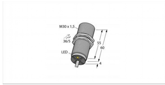
BI10-M30-AP6X, M30 (10 mm føleavstand)
